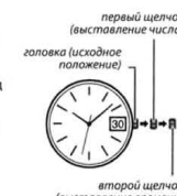
второй щелчок (выставление времени)
